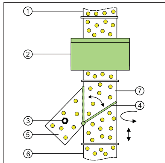
1) Entrée du produit 2) Bobine de détection 3) Pièce métallique 4) Volet éjecteur 5) Sortie des rejets 6) Sortie du produit contrôlé 7) Unité d'éjection (orientable et déplaçable)
